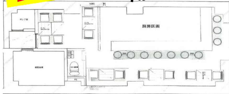
※イメージ平面図 (11.36坪 22席)
